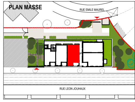
PLAN ECHELLE 1/80
